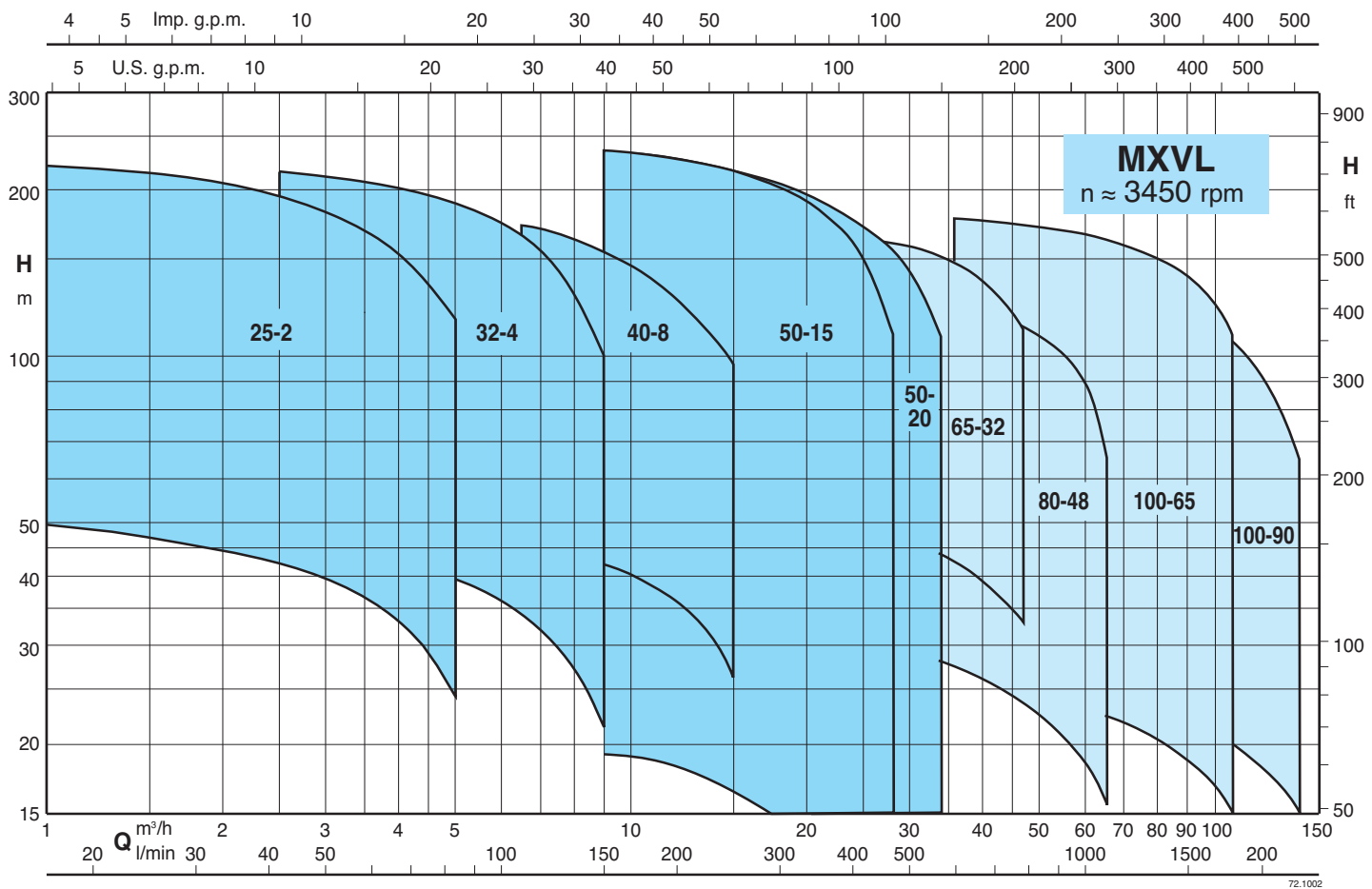
Coverage chart - Campo de aplicaciones n ≈ 3450 rpm
